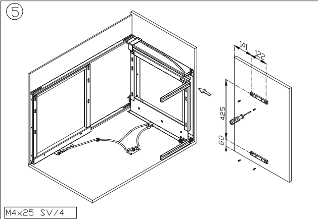
M4x25 SV/4
