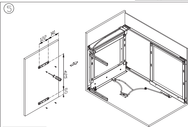
M4x25 SV/4
